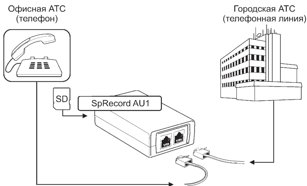
Рисунок 2.1 Схема подключения адаптера SpRecord AU1
